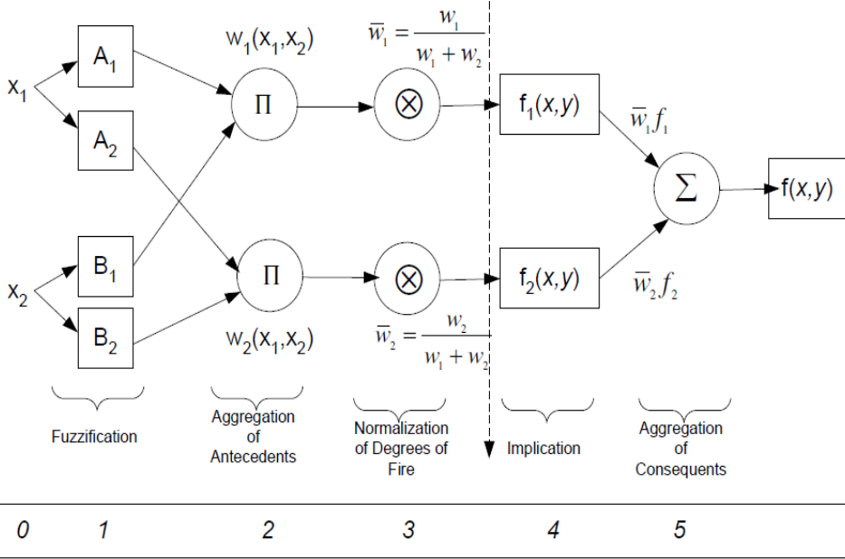
Şekil 9. 2 girdili ve 2 kurallı Sugeno tipi bulanık çıkarıma eşdeğer ANFIS mimarisi
